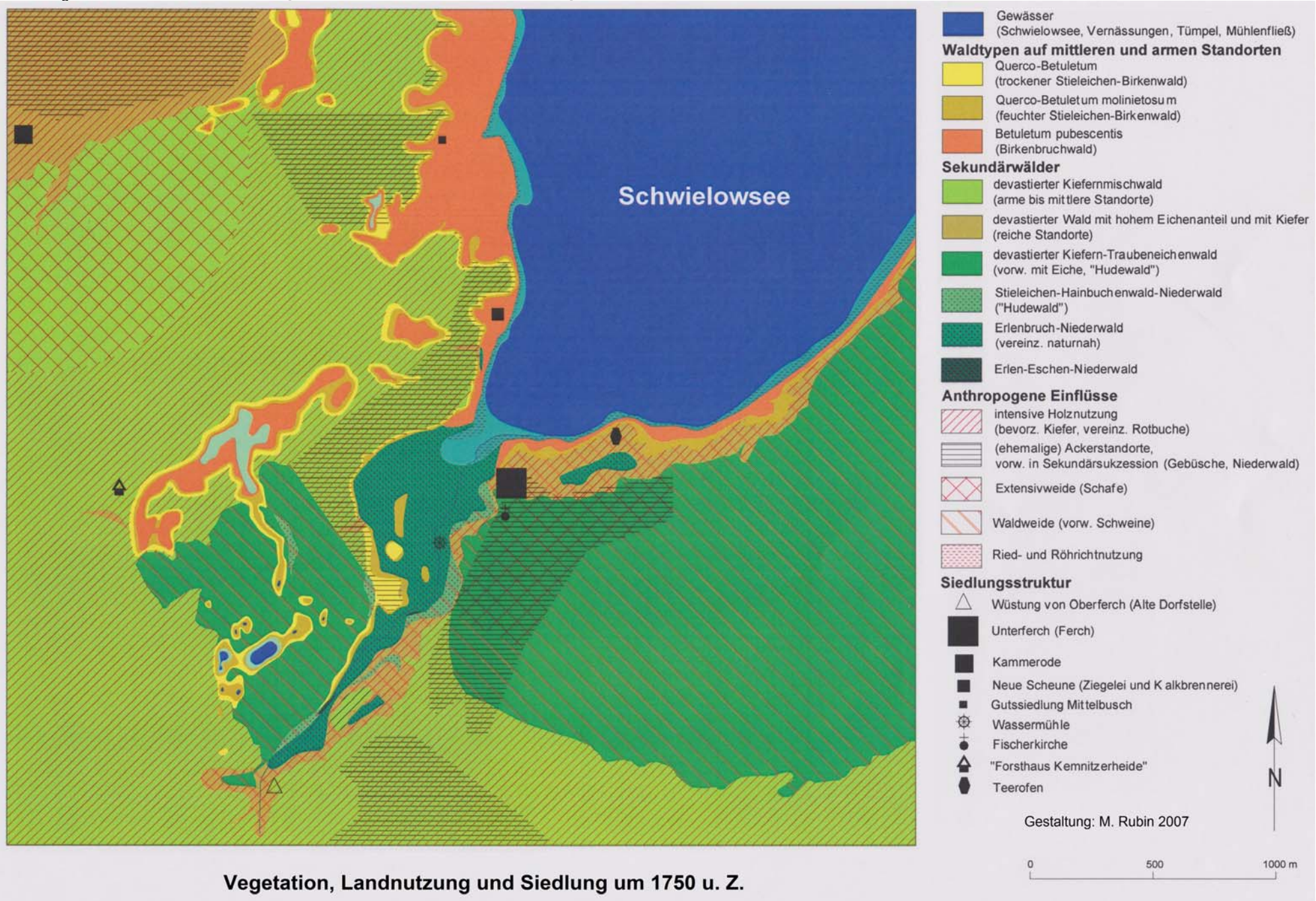
Abbildung 13: Waldzustand um 1750 u. Z. [aus Rubin, M., Brande, A. & Zerbe, S. 2008]
