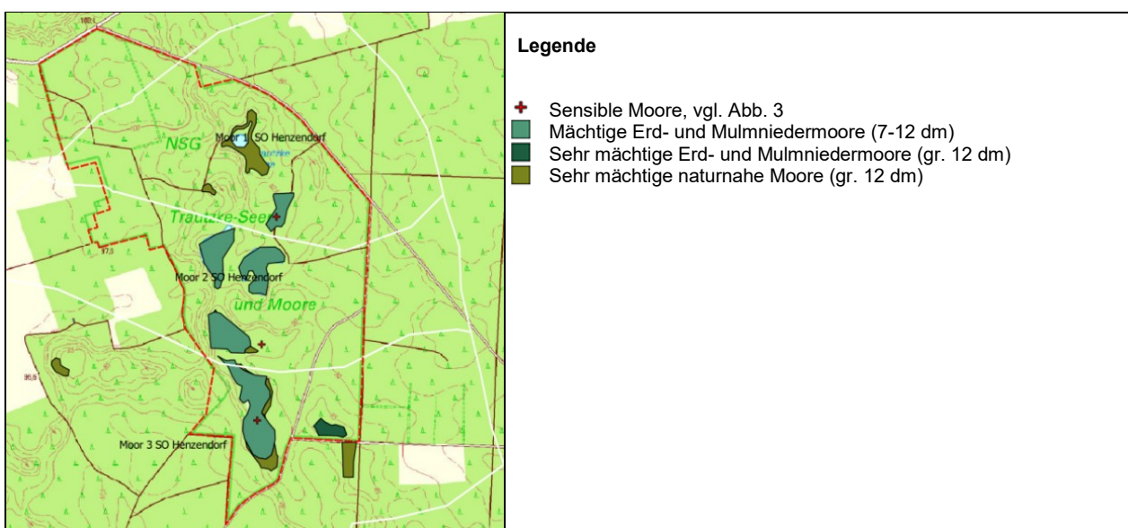
Abb. 4: Moorbodenformen im FFH-Gebiet Trautzke-Seen und Moore (Quelle: MoorFIS 2014, LBGR)
