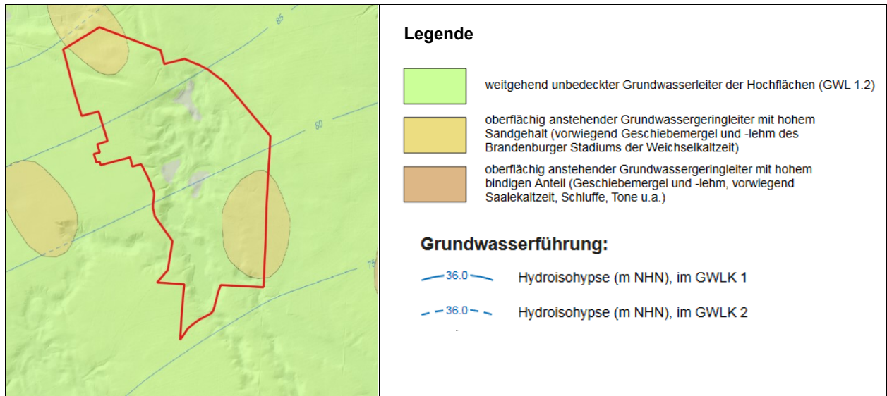
Abb. 5: Ausschnitt aus der hydrogeologischen Karte 1:50.000 (HYK 50-1, LBGR 2014) im Bereich des FFH-Gebietes Trautzke-Seen und Moore
