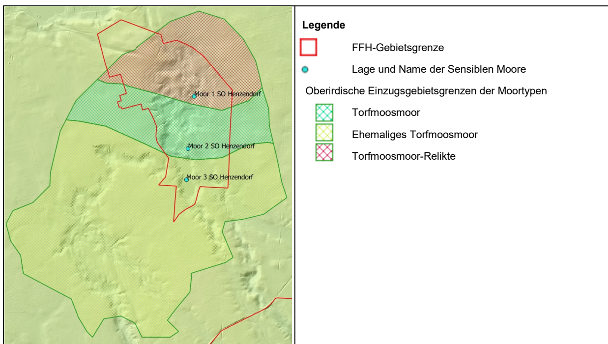
Abb. 3: Oberirdische Einzugsgebiete der drei als sensible Moore eingestuft Moore im FFH-Gebietes Trautzke-Seen und Moore (LUA 2009)
