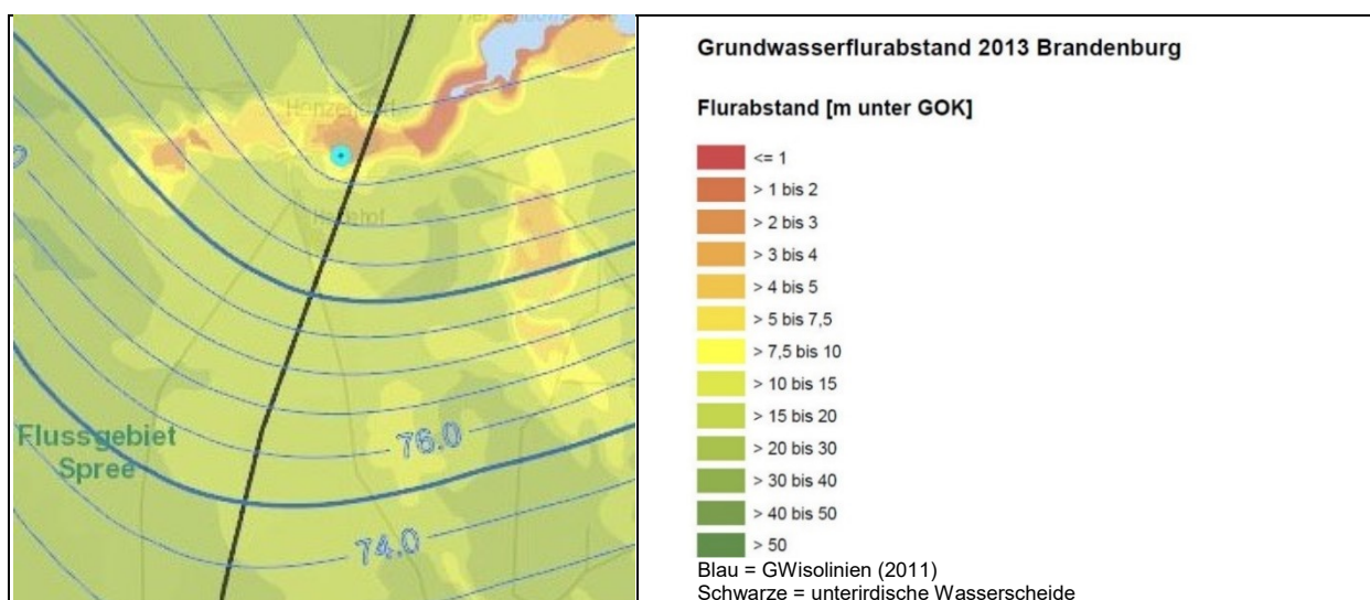
Abb. 6: Grundwasserisolinien und -flurabstand im Bereich des FFH-Gebietes Trautzke-Seen und Moore (Meßstelle Henzendorf, Datenerhebung 2011, LfU)
