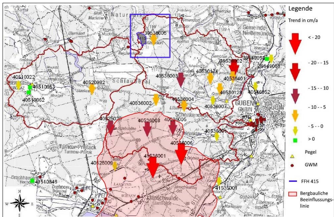
Abb. 7: Entwicklung der Grundwasserstände im großräumigen Umfeld des FFH-Gebietes Trautzke-Seen und Moore (2000 – 2010 aus TSCHIRSCHNITZ & PURZ 2010) und die Lage der Bergbaulichen Beeinflussungslinie im Jahr 2020 (LEAG 2019), ergänzt
