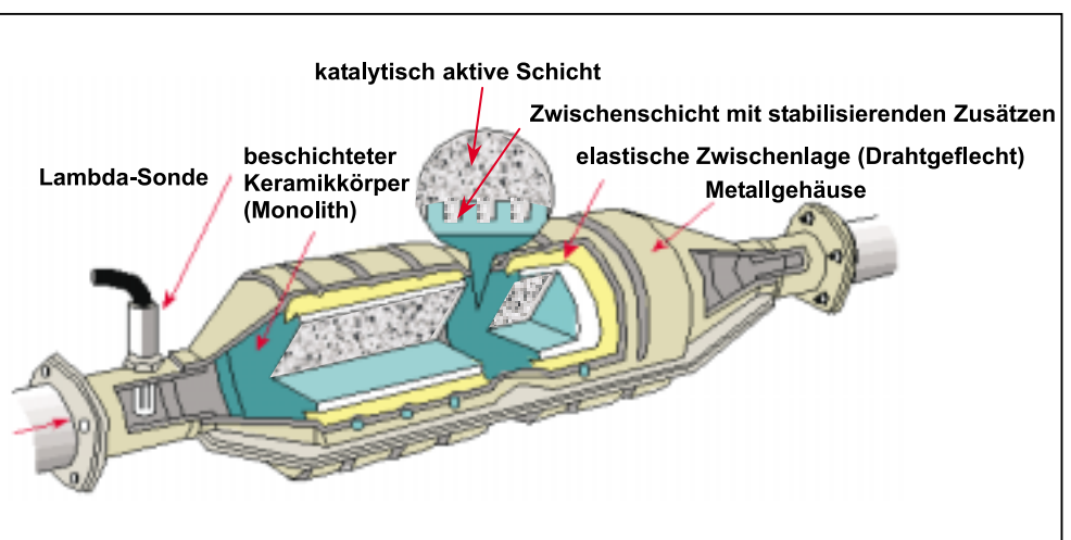
Abb. 2: Schema eines Drei-Wege-Katalysators für Ottomotoren mit Aufbau der Katalysatorschicht (ROMPP 1995)
