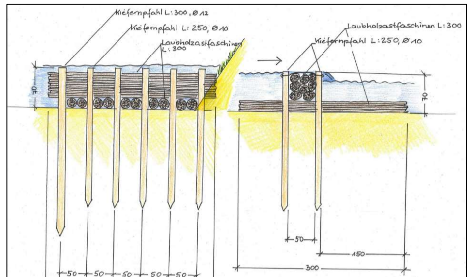
Ausführungszeichnungen: links Längsschnitt, rechts Querschnitt
