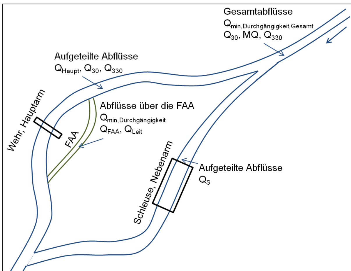
Abbildung 2-2: Übersichtsschema der verwendeten Abflussbegriffe
