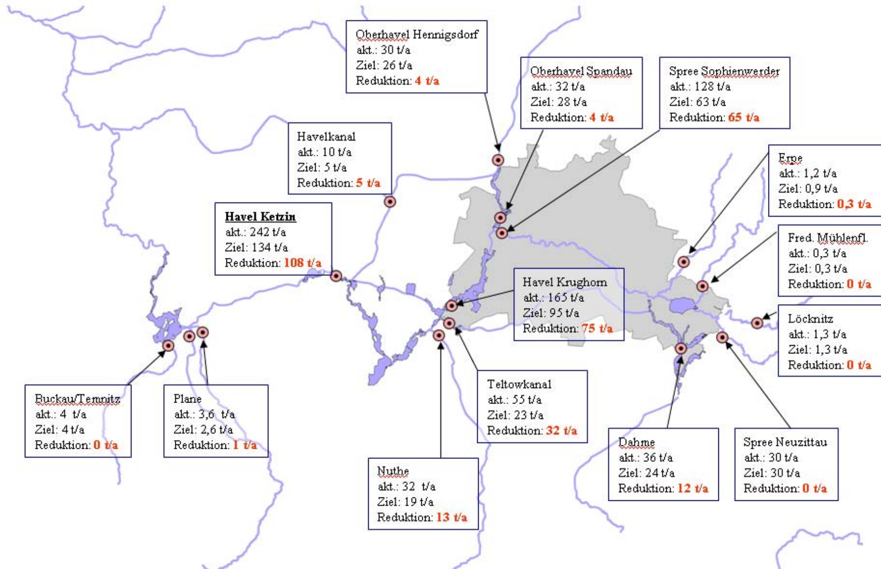
Abb. IV-3: Aktuelle Frachten (Mittel 2007-2009), Zielfrachten und Reduktion für Gesamt-Phosphor an den Bilanzpegeln.
