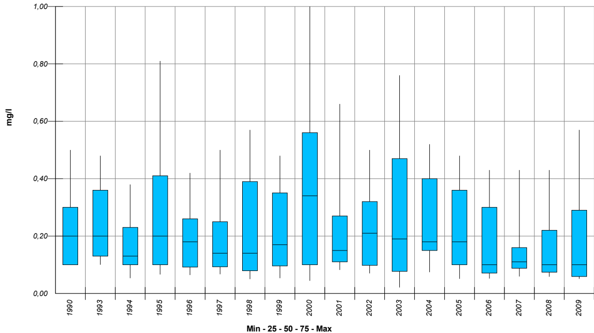
Abb. IV-2: Langzeitentwicklung der Gesamtposphorkonzentration in der Havel im Abstrom der Metropolenregion Berlin (Pegel Havel, Krughorn)
