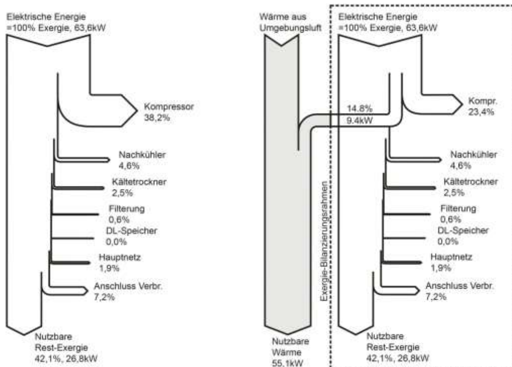
A.5-6: Exergieverluste in einer beispielhaften herkömmlichen pneumatischen Anwendung, Fortführung aus Abbildung A.5-5
