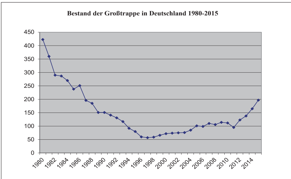
Abb. 5: Bestandsentwicklung der Großtrappe in Deutschland 1980 bis 2015.
